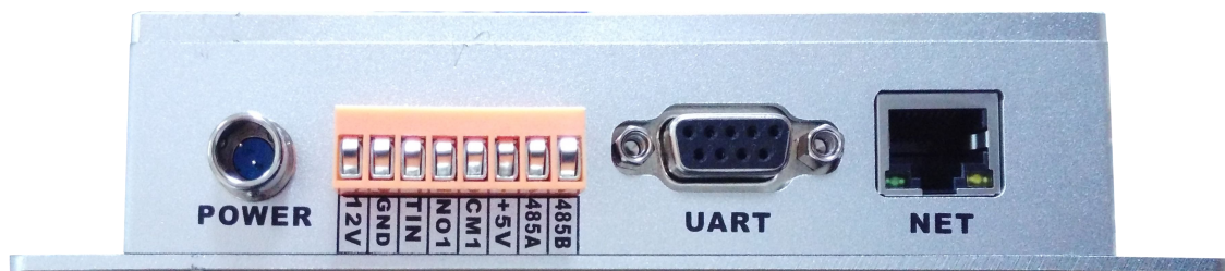
图 2 JT-9230 读写器外形图
